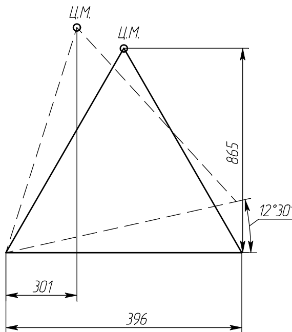
Рисунок 1 - Схема устойчивости агрегата Д 6300-80-2.
